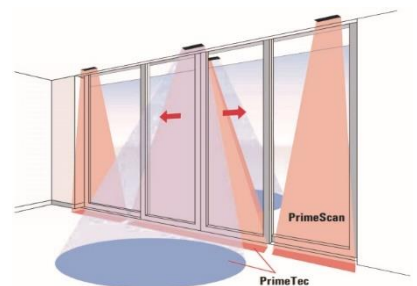
In dieser Abbildung ist eine Schiebetür mit den Absicherungs-(rot) und Aktivierungsfelder (blau) zu sehen. Um die funktionale Sicherheit zu gewährleisten, müssen die Türsensoren die Haupt- und Nebenschliesskante absichern.
