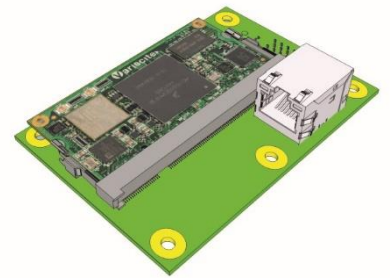
Zukünftige Bircher Reglomat Sensoren könnten mit einem integrierten Zusatzmodul als Gateway agieren. Eine mögliche Variante, wie ein solches Zusatzmodul aussehen könnte, ist in der Abbildung oberhalb modelliert.
