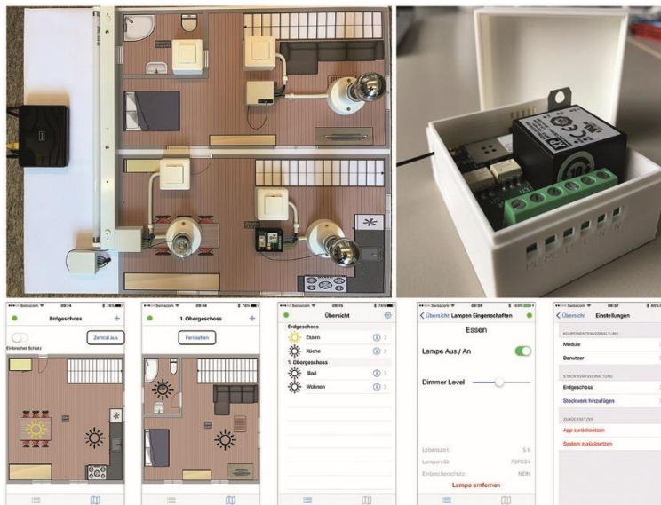
Das Bild zeigt den Demonstrationaufbau (oben links), ein einzelnes Smart Light Modul (oben rechts) und die Smart Light App (unten).
